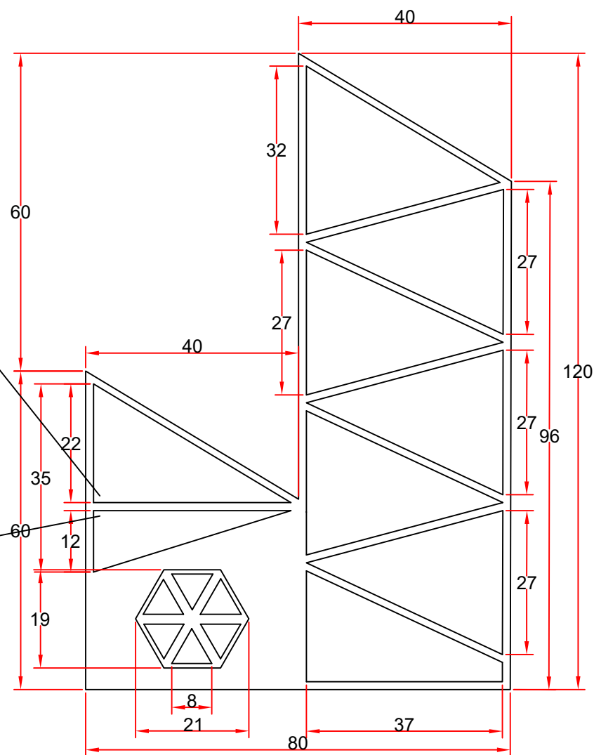
TAMPAK DEPAN
